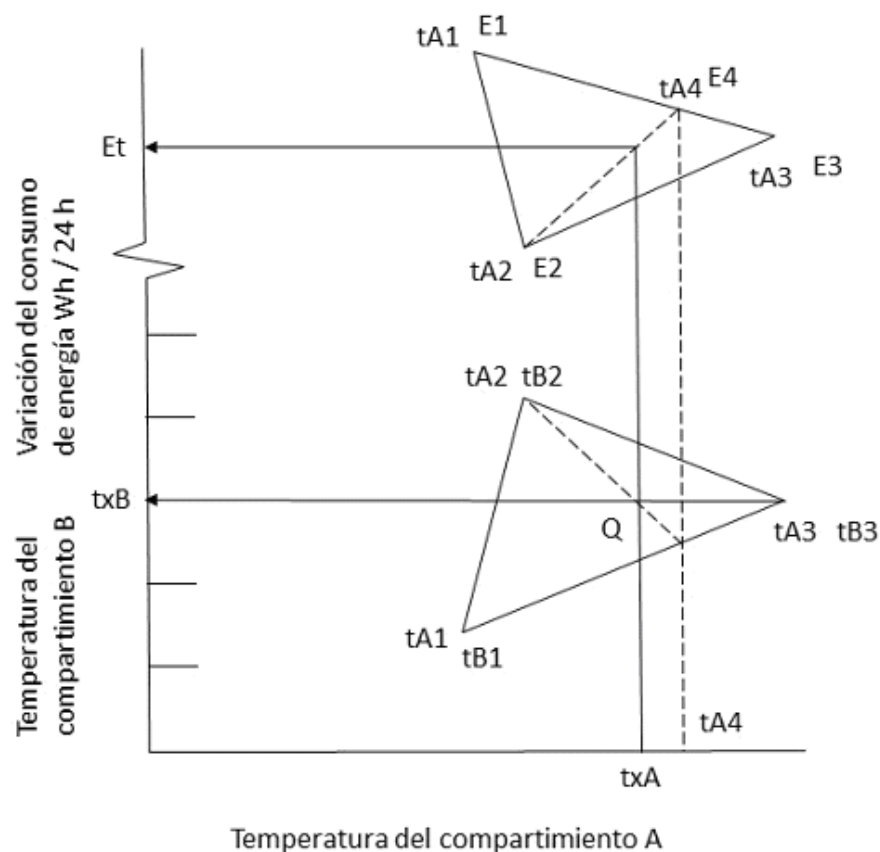
Figura D.1-Ejemplo gráfico para un aparato de refrigeración con múltiples compartimentos con dos o más controles que regulan la temperatura de los compartimentos-dos controles ajustados.
