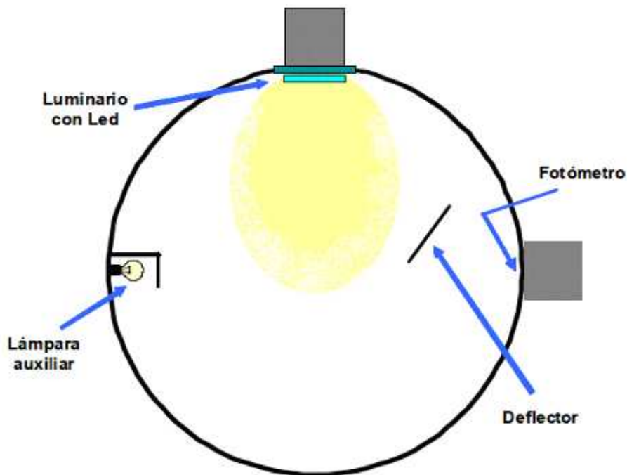
Figura F2. Configuración de la esfera integradora 2T
