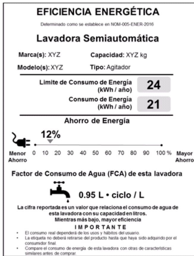
Figura 3 Ejemplo de distribución de la información de la etiqueta de lavadoras de ropa electrodomésticas semiautomáticas
