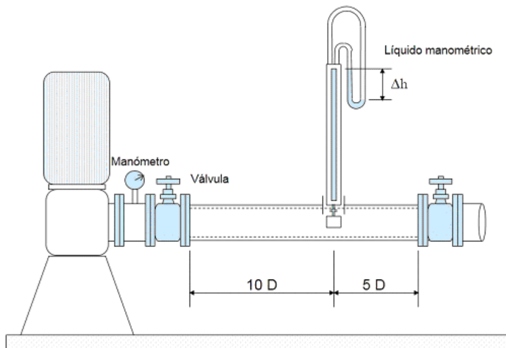
Figura 1.- Medición de flujo con tubo de Pitot.
