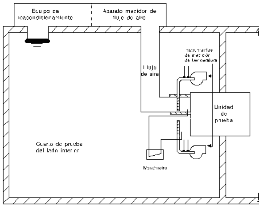
FIGURA 5. Aparato de medición de flujo de aire
