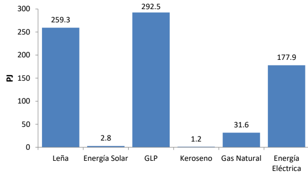
Gráfica 4.9 Principales combustibles usados en el sector doméstico en México, 2010
