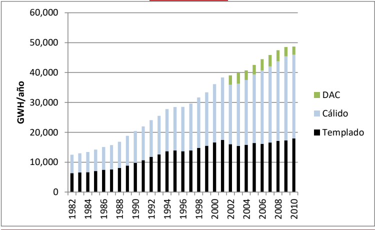
Gráfica 4.11. Evolución del consumo de energía eléctrica del sector residencial de México (1982 a 2010) 5
