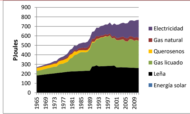
Gráfica 4.9 . Consumo de energía del sector residencial 1965-2010
