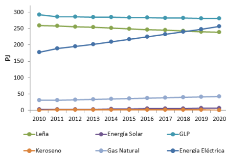
Gráfica 4.130 Tendencia de crecimiento del consumo de energía en el sector residencial (2010-2020)
