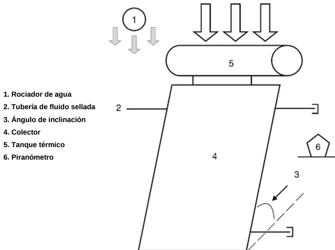
Figura A.6-Penetración por lluvia
