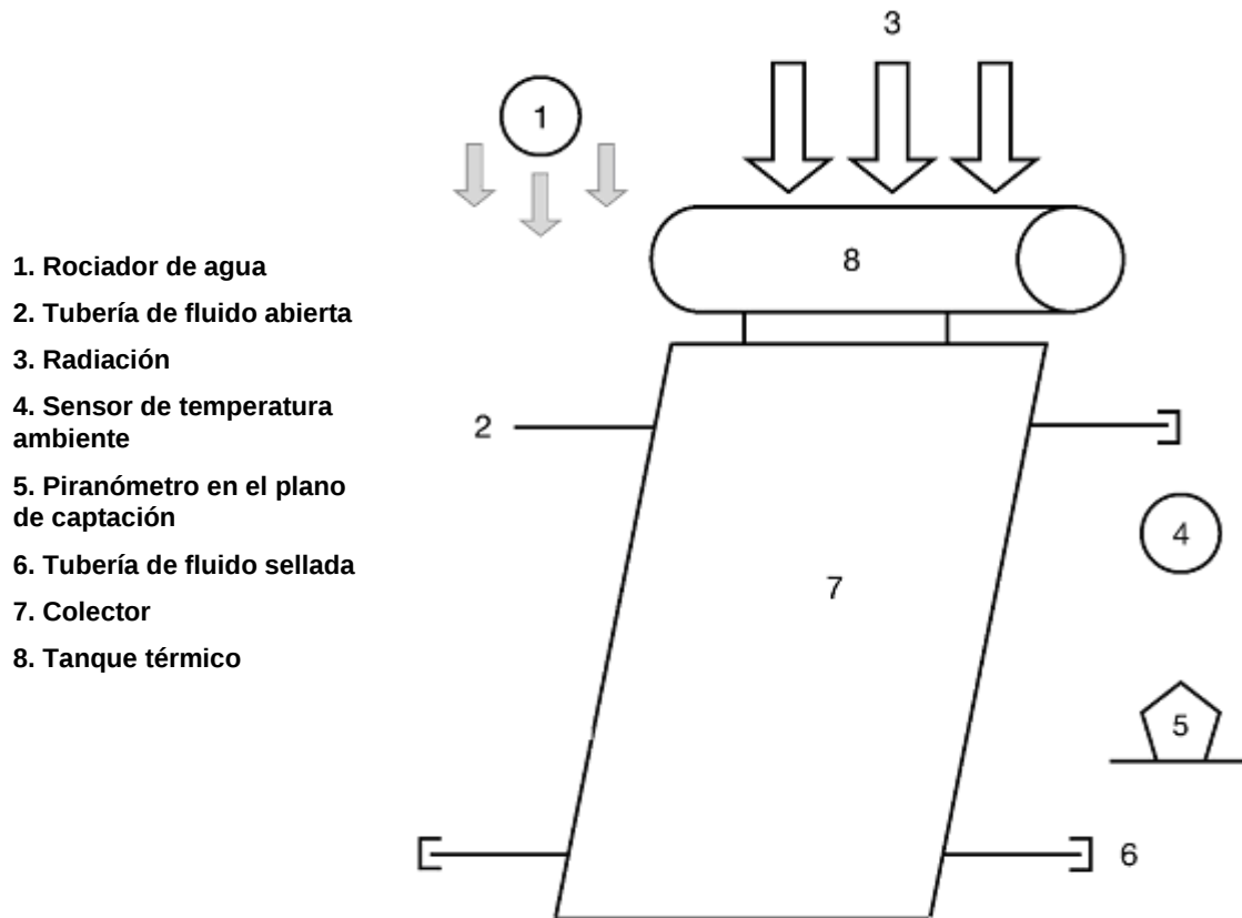
Figura A.5-Choque térmico externo
