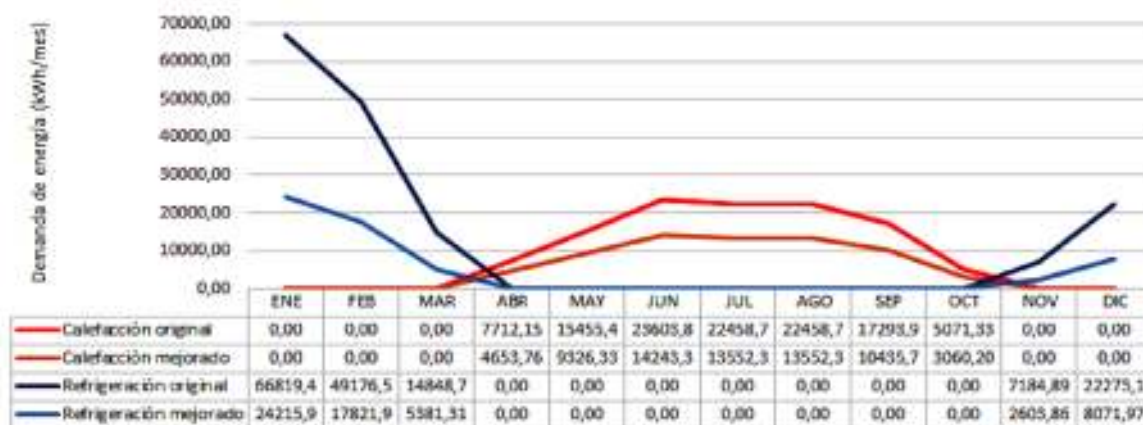
Figura 1 - Comparación anual de la variación de demanda de energía simulada del caso original y mejorado. Municipalidad de Rauch.
