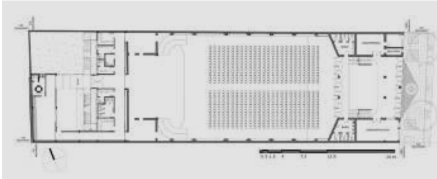
Figura 45 - Planta baja Cine Teatro Plaza, ubicado en Godoy Cruz, provincia de Mendoza
